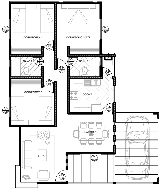
PLANTA DE ARQUITECTURA
