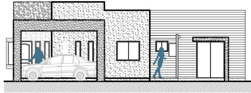
ELEVACION LATERAL DERECHA
