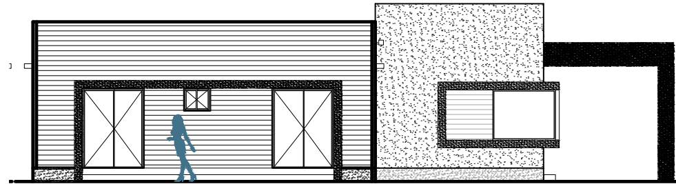
ELEVACION LATERAL IZQUIERDA
