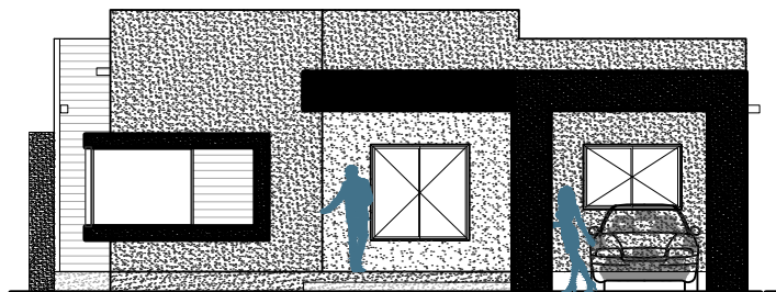
ELEVACION PRINCIPAL
