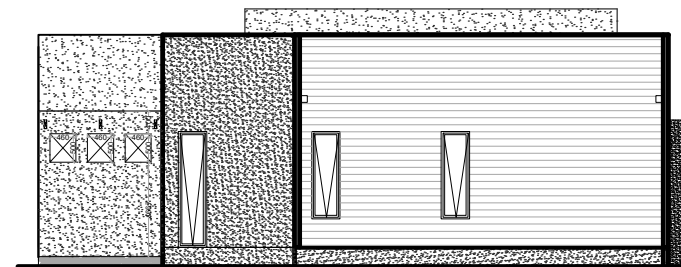
ELEVACION POSTERIOR
